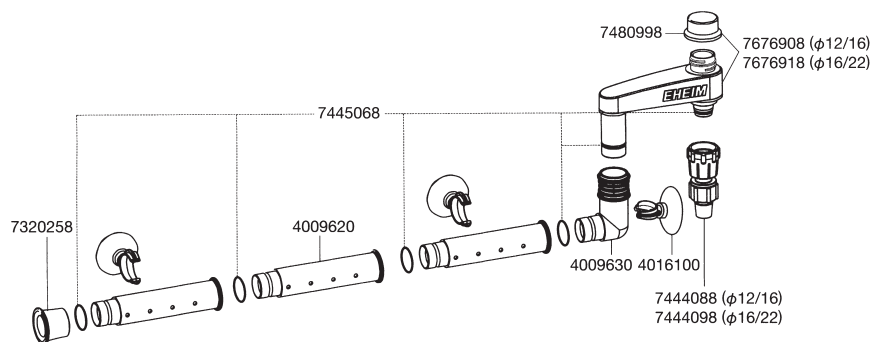
エーハイムインスレーションセット2 (排水) 用パーツ
